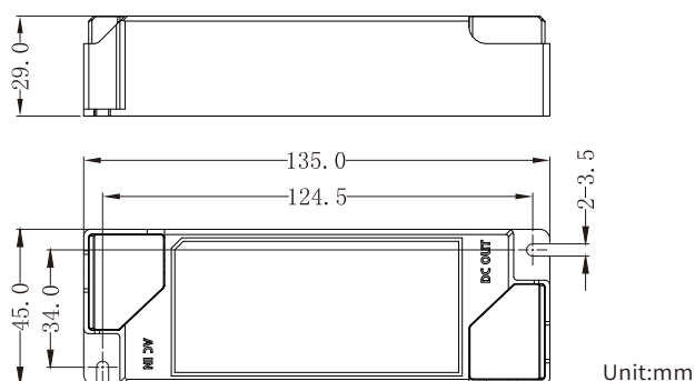
BK-PQL042/PQL050
